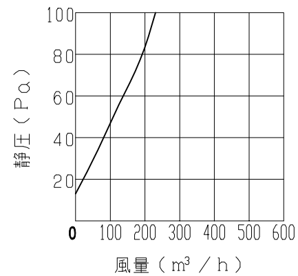
圧力損失曲線
